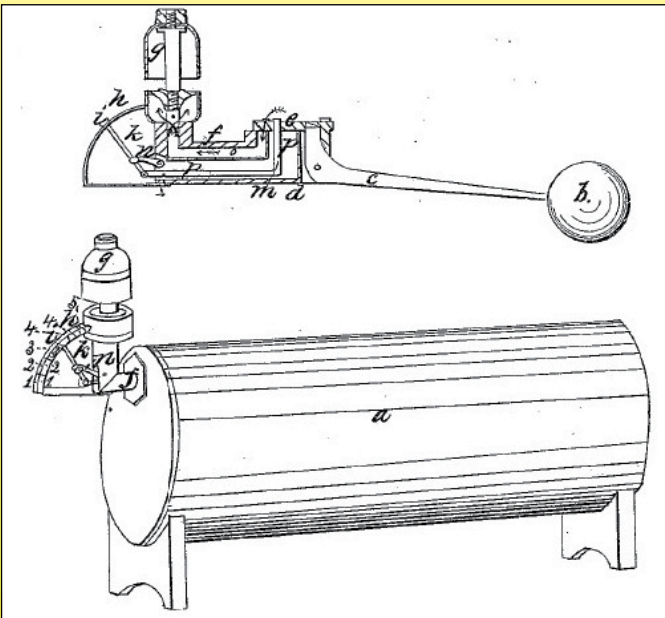
Джозеф Дилкс, патент США 7808, декабрь 1850 года, поплавковый индикатор уровня с паровым сигнальным свистком.
